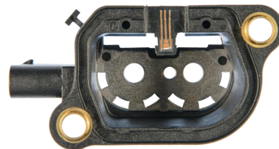
Hallsensor: Laserschweißen und Direktumspritzung
